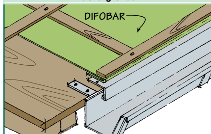
Fissaggio di DIFOBAR in corrispondenza della gronda
