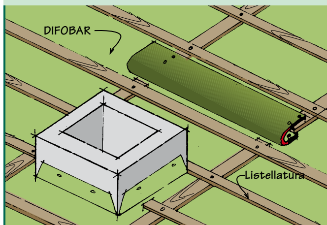
4. Posa della listellatura e fissaggio della fascia aggiuntiva di DIFOBAR
