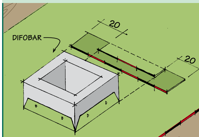
2. Posizionamento fascia aggiuntiva di DIFOBAR
