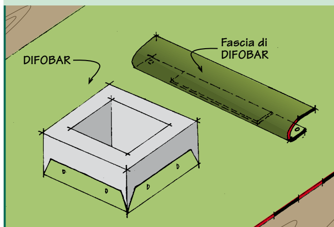
3. Piegatura fascia di DIFOBAR
