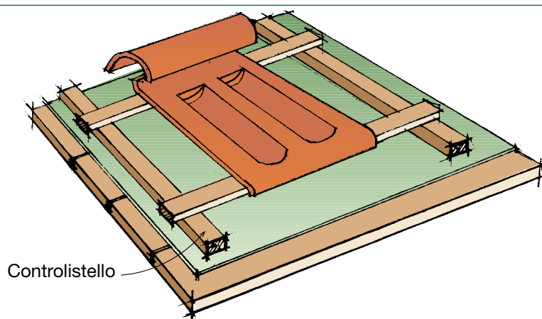
Fogli sottotegola fissati paralleli alla linea di gronda
