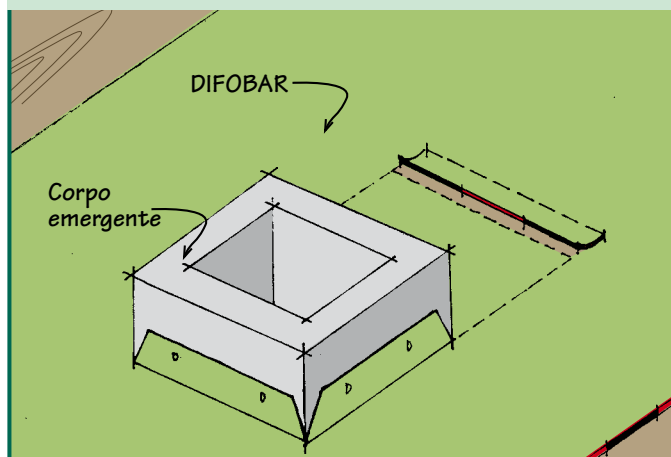
1. Incisione di DIFOBAR a monte del corpo emergente
